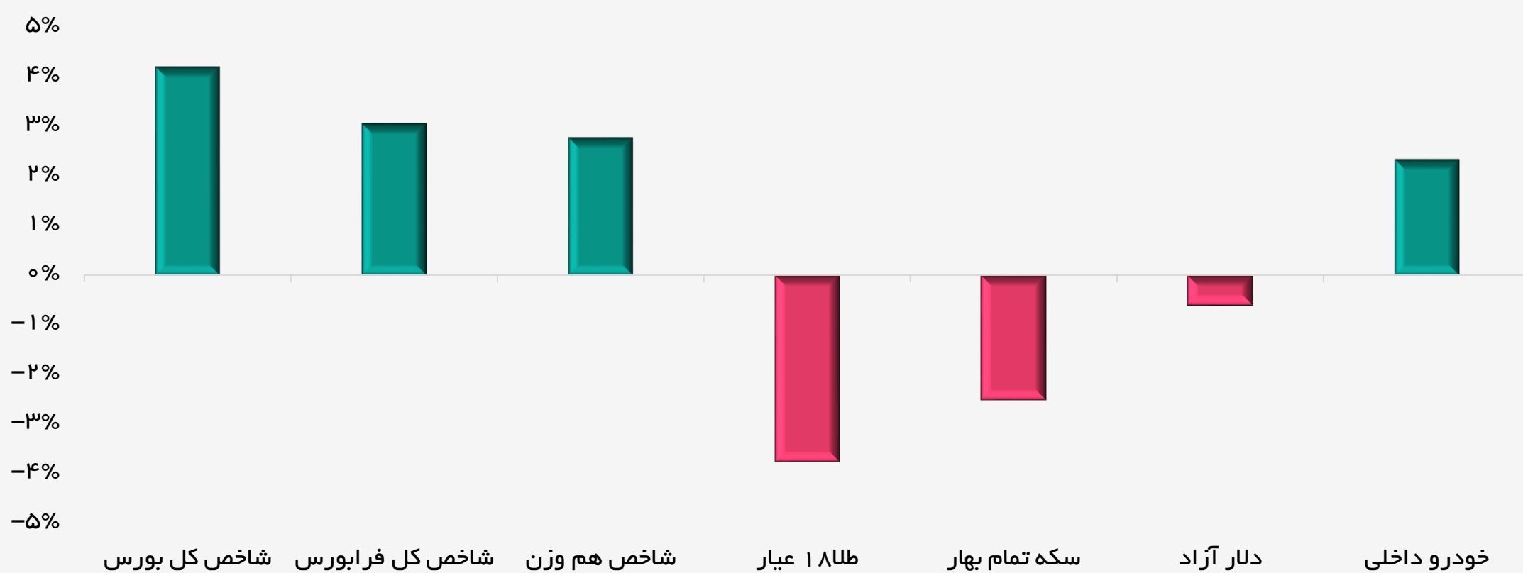
بازدهی هفتگی
